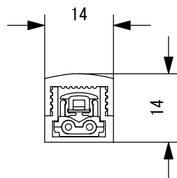
断面寸法図 2/1
