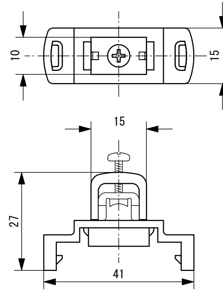
ワイヤーロック部寸法図
