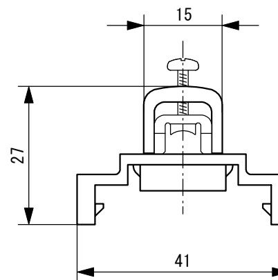
ワイヤーロック部寸法図
