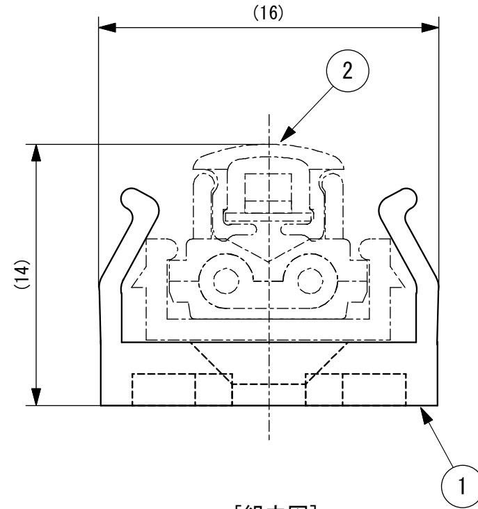
[組立図]
