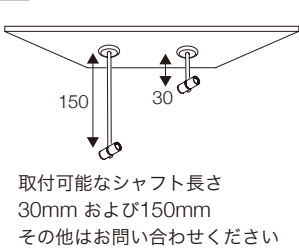
図3 天付け施工
