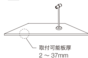
図2 平置き施工
